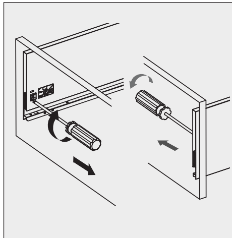
Réglage latéral \pm 2 mm Lateral adjustment \pm 2 mm
