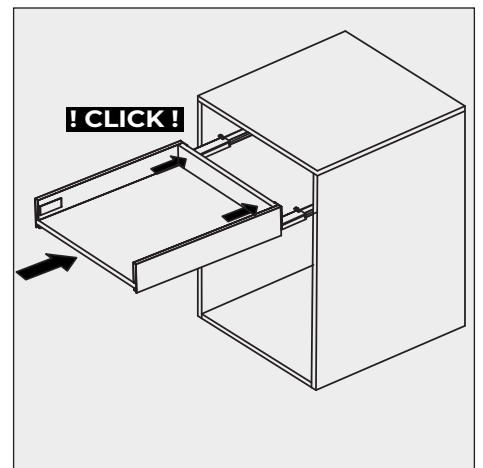
Refermer complètement pour clipser sur les coulisses. Slide the drawer all the way in and close completely to clip on the slides.
